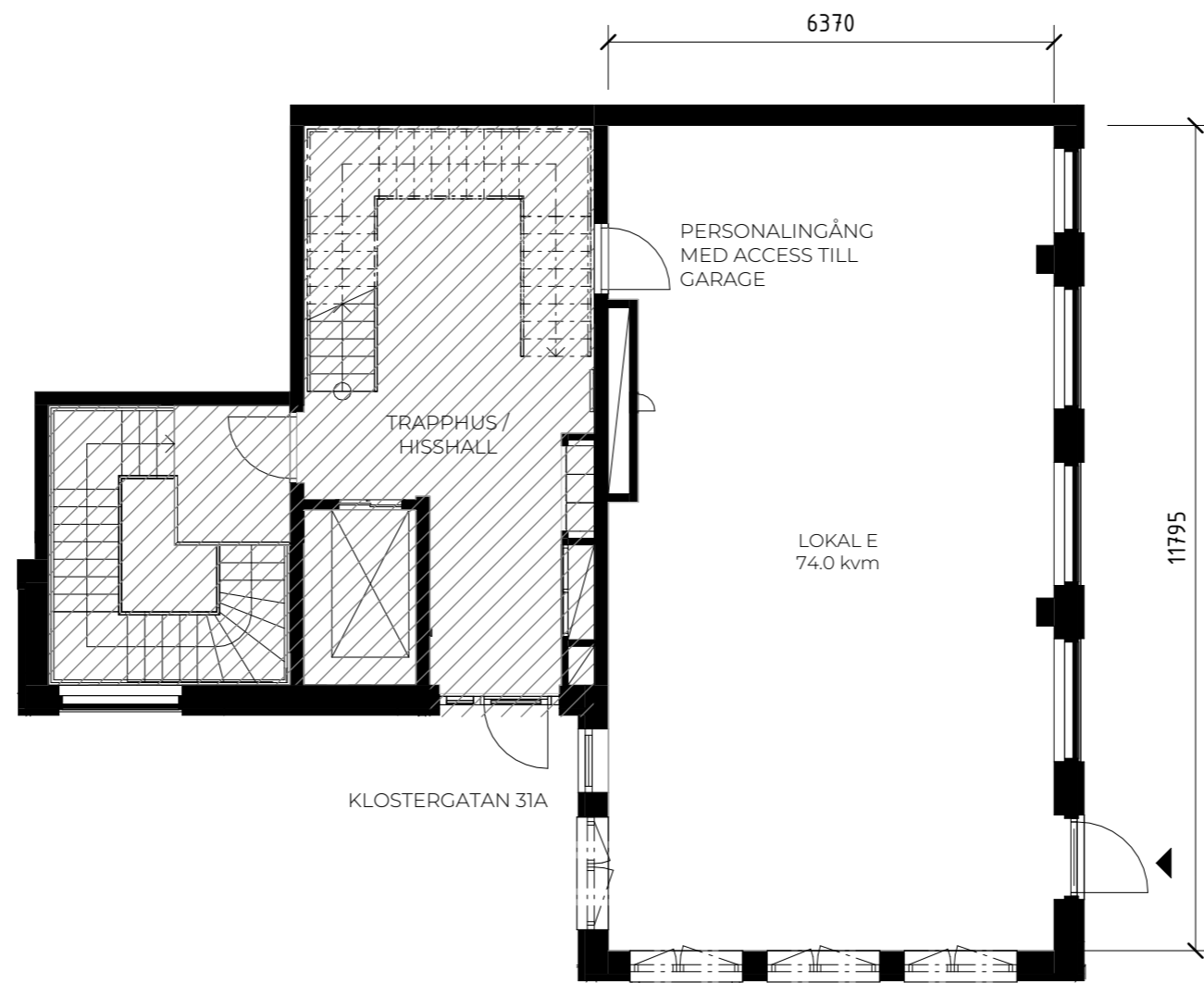
LOKAL E SKALA 1 : 100
